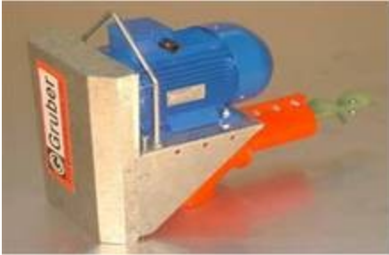
Pogon preko klinastog remena sa kaišom, i koturom
